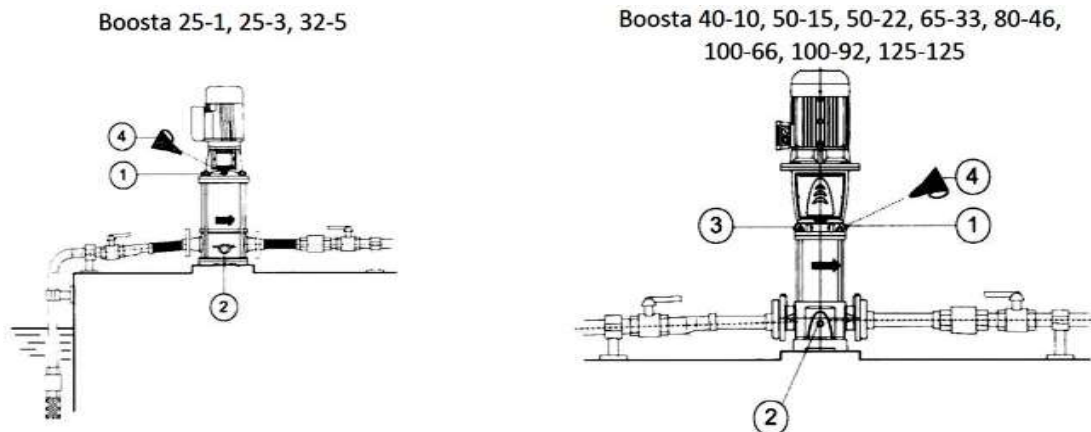
Рисунок 8 – Установки насоса выше уровня перекачиваемой жидкости
