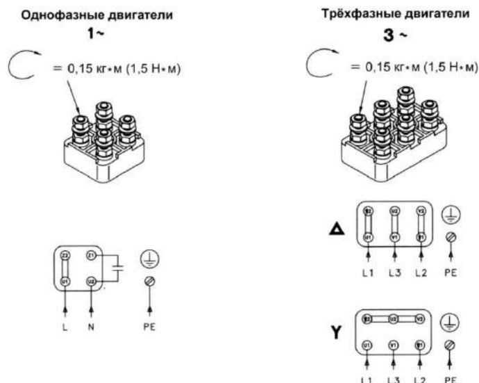
Рисунок 4 – Электрическая схема
