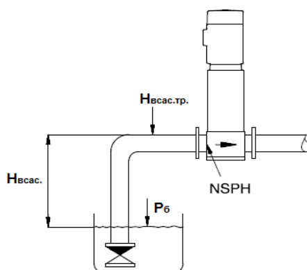
Рисунок 1 – Высота всасывания
