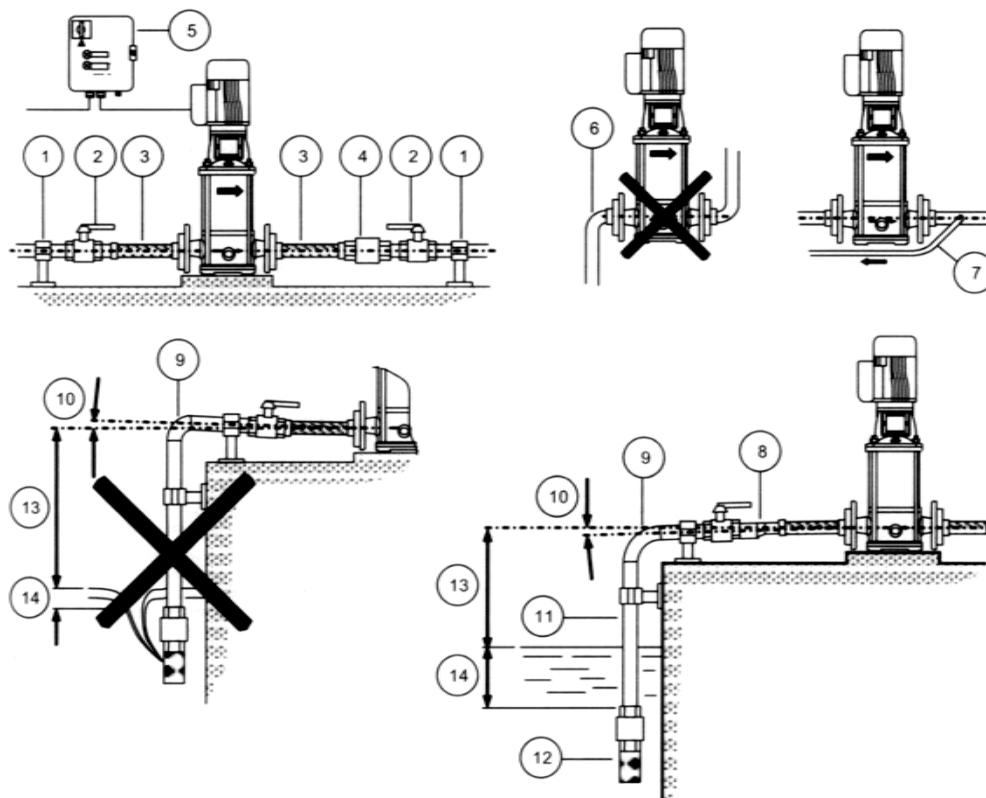
Рисунок 2 – Схема монтажа
