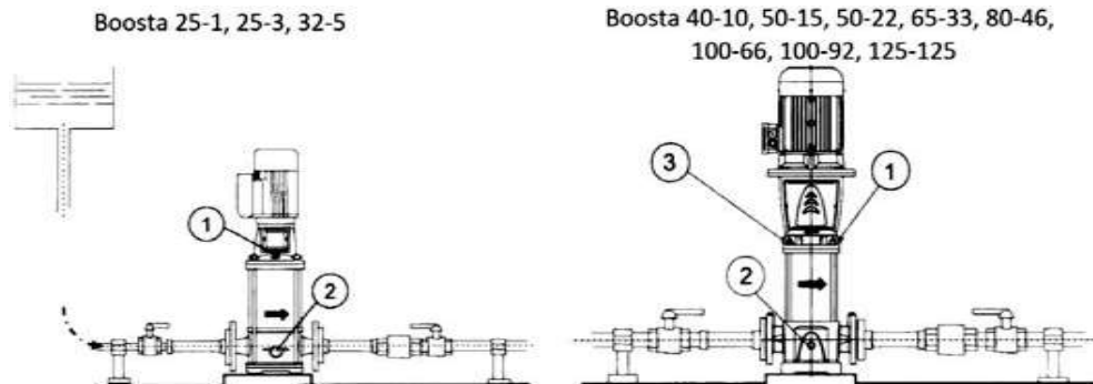
Рисунок 7 – Установки насоса ниже уровня перекачиваемой жидкости
