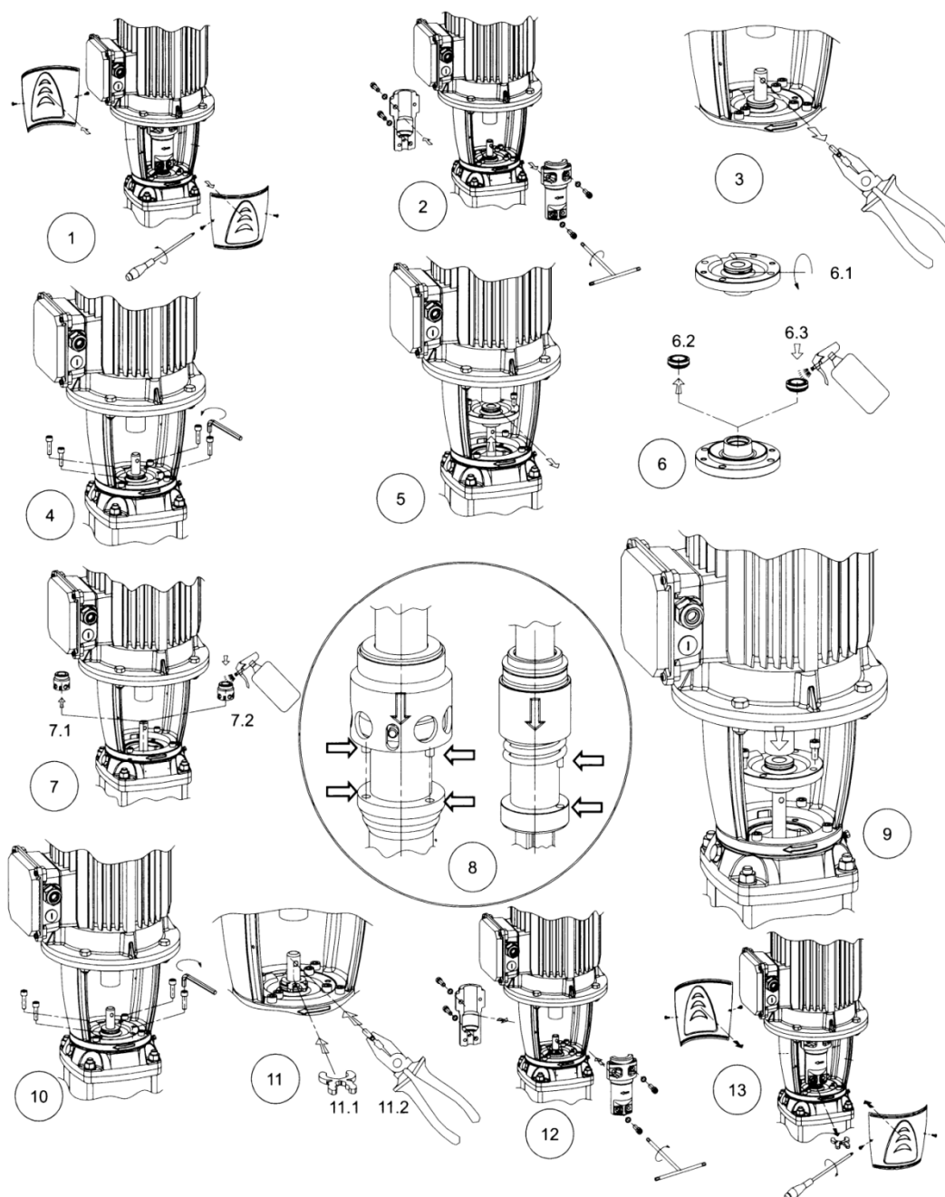
Рисунок 10 – Замена (установка) торцового уплотнения
