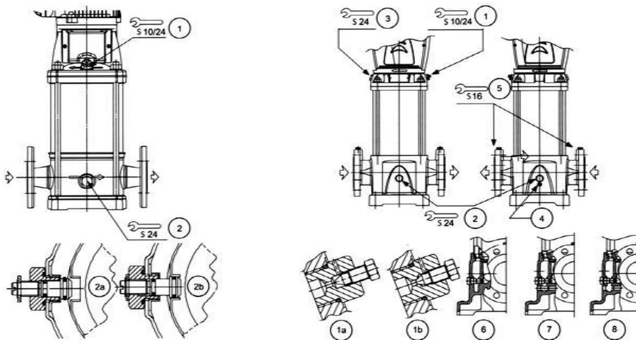
Рисунок 6 – Назначение пробок в насосе
