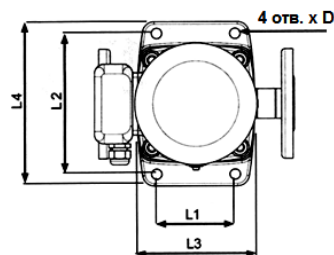
Рисунок 3 – Размеры для установки
