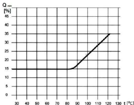
Рисунок 5 – Минимальные значения подачи
