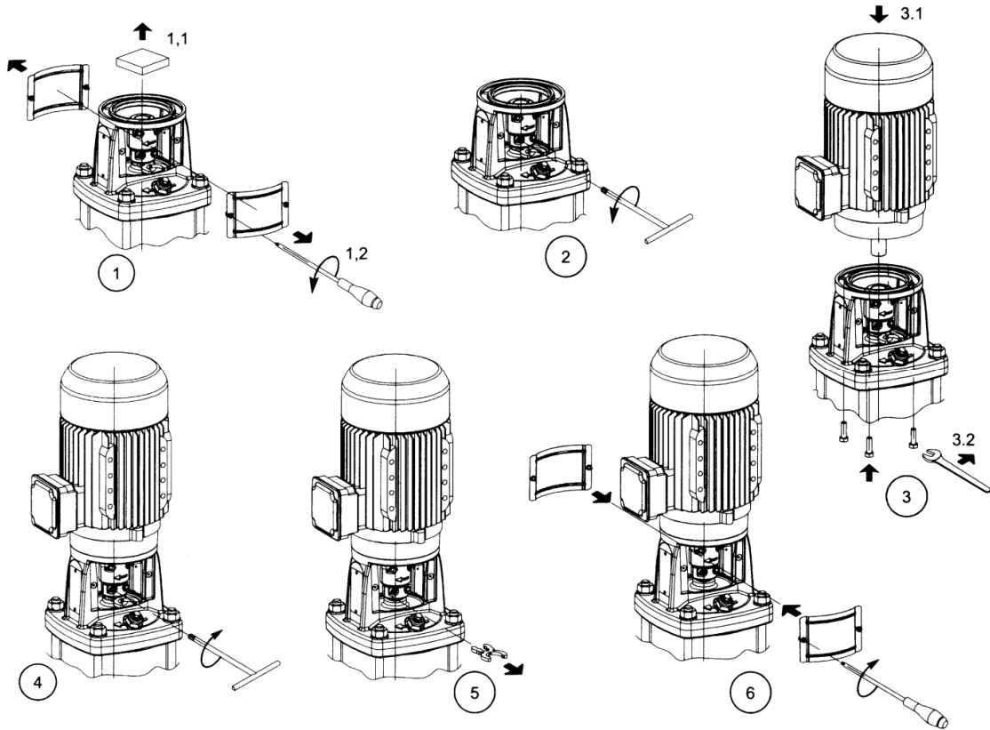
Рисунок 9 – Замена (установка) двигателя
