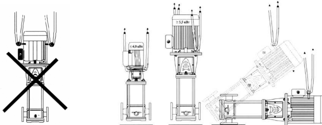
Рисунок 11 – Строповка насоса с двигателем
